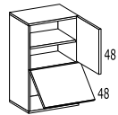
PENSILE DX O SX 1 anta – 1 anta vasistas 2 ripiani
