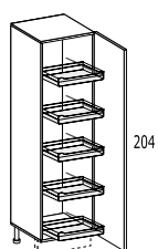
COLONNA DX O SX CON MECCANISMO CESTI ESTRAIBILI 1 anta
