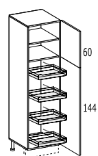
COLONNA DX O SX CON MECCANISMO CESTI ESTRAIBILI 2 ante – 1 ripiano
