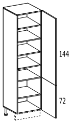
COLONNA DX O SX 2 ante – 5 ripiani
