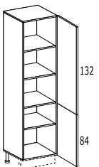
COLONNA DX O SX 2 ante – 4 ripiani
