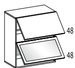
PENSILE VASISTAS (FUSTO INTERO) 1 anta – 1 anta vetro 1 ripiano – 1 ripiano cristallo
