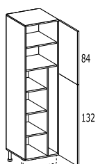
COLONNA PORTASCOPE DX O SX 2 ante - 1 tramezza - 4 ripiani
