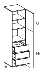
COLONNA DX O SX 2 ante c/cerniere 180° 2 ripiani + 3 cestoni interni
