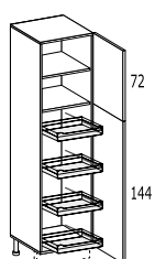
COLONNA DX O SX CON MECCANISMO CESTI ESTRAIBILI 2 ante - 1 ripiano
