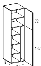
COLONNA PORTASCOPE DX O SX 2 ante - 1 tramezza - 4 ripiani
