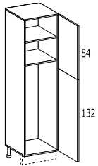
COLONNA PORTASCOPE DX O SX 2 ante - 1 ripiano fisso h.160 - 1 ripiano
