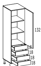
COLONNA DX O SX 1 anta – 4 cassetti – 2 ripiani
