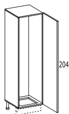
COLONNA DX O SX PER FRIGORIFERO 1 ante
