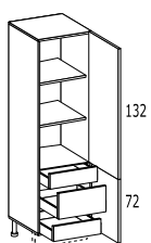
COLONNA DX O SX 2 ante c/cerniere 180° – 2 ripiani – 2 cassetti + 1 cestone interni
